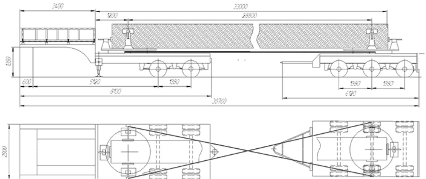
Автопоезд специализированный (рабочее положение с грузом)
